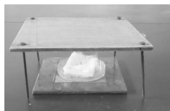
図1 トラップの模式図 (上) 屋外試験で用いたトラップ (下)
