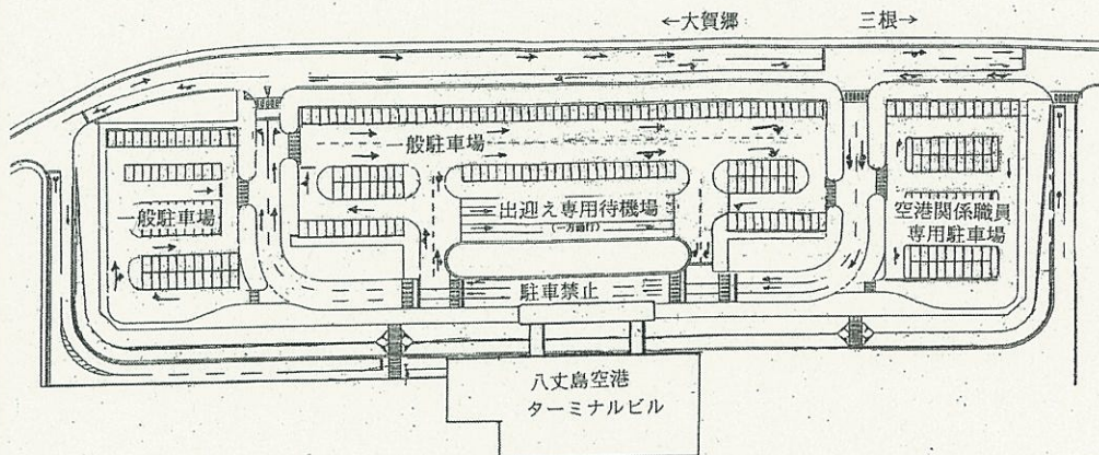
八丈島空港駐車場平面図
